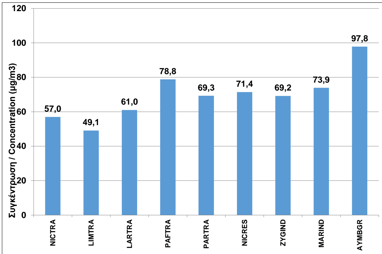
Σχήμα 7: Ετήσιοι μέσοι όροι O 3 στους Σταθμούς Παρακολούθησης Ποιότητας Αέρα για το έτος 2018. Figure 7: O 3 annual mean concentration in Air Quality Monitoring Stations for the year 2018.
