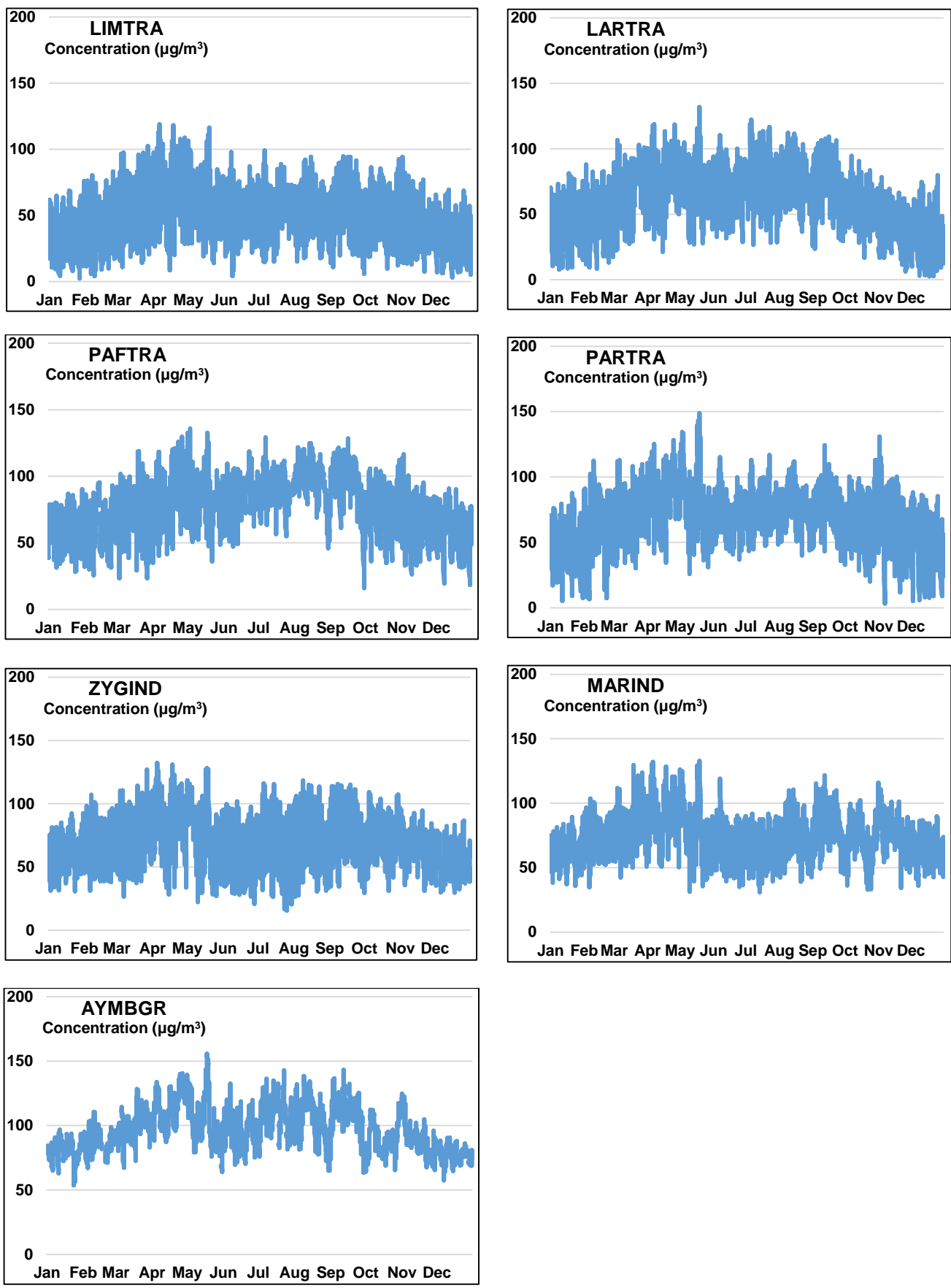
Σχήμα 8: Μέσες 8-ωρες τιμές όζοντος (O 3 ) στους Σταθμούς Παρακολούθησης Ποιότητας Αέρα για το έτος 2018 (Μέγιστος ημερήσιος μέσος όρος οκταώρου – Τιμή Στόχος: 120 µg/m 3 ).
