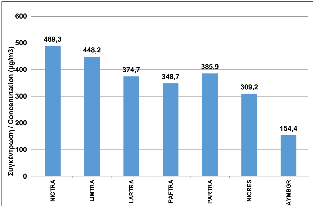
Σχήμα 9: Ετήσιοι μέσοι όροι CO στους Σταθμούς Παρακολούθησης Ποιότητας Αέρα για το έτος 2018. Figure 9: CO annual mean concentration in Air Quality Monitoring Stations for the year 2018.
