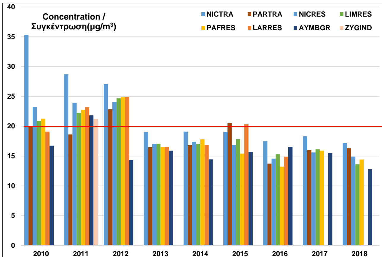
Σχήμα 13: Ετήσιοι μέσοι όροι ΑΣ 2.5 στους Σταθμούς Παρακολούθησης Ποιότητας Αέρα για την περίοδο 2010-2018 (Ετήσια οριακή τιμή: 20 µg/m 3 ).
