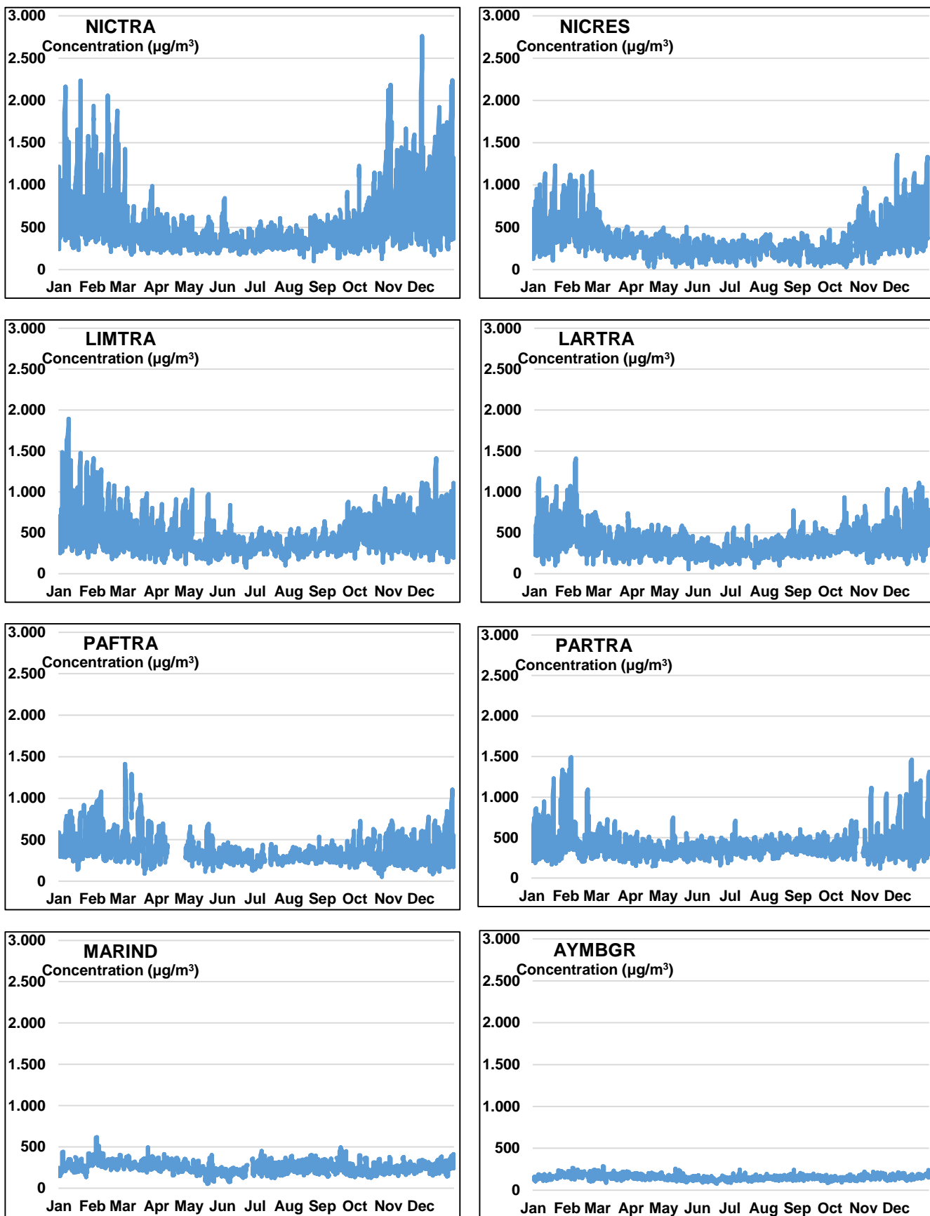
Σχήμα 10: Μέσες 8-ωρες τιμές μονοξειδίου του άνθρακα (CO) στους Σταθμούς Παρακολούθησης Ποιότητας Αέρα για το έτος 2018 (Οριακή Τιμή μέγιστου ημερήσιου μέσου όρου οκταώρου: 10.000 \mu\text{g}/\text{m}^3 ).
