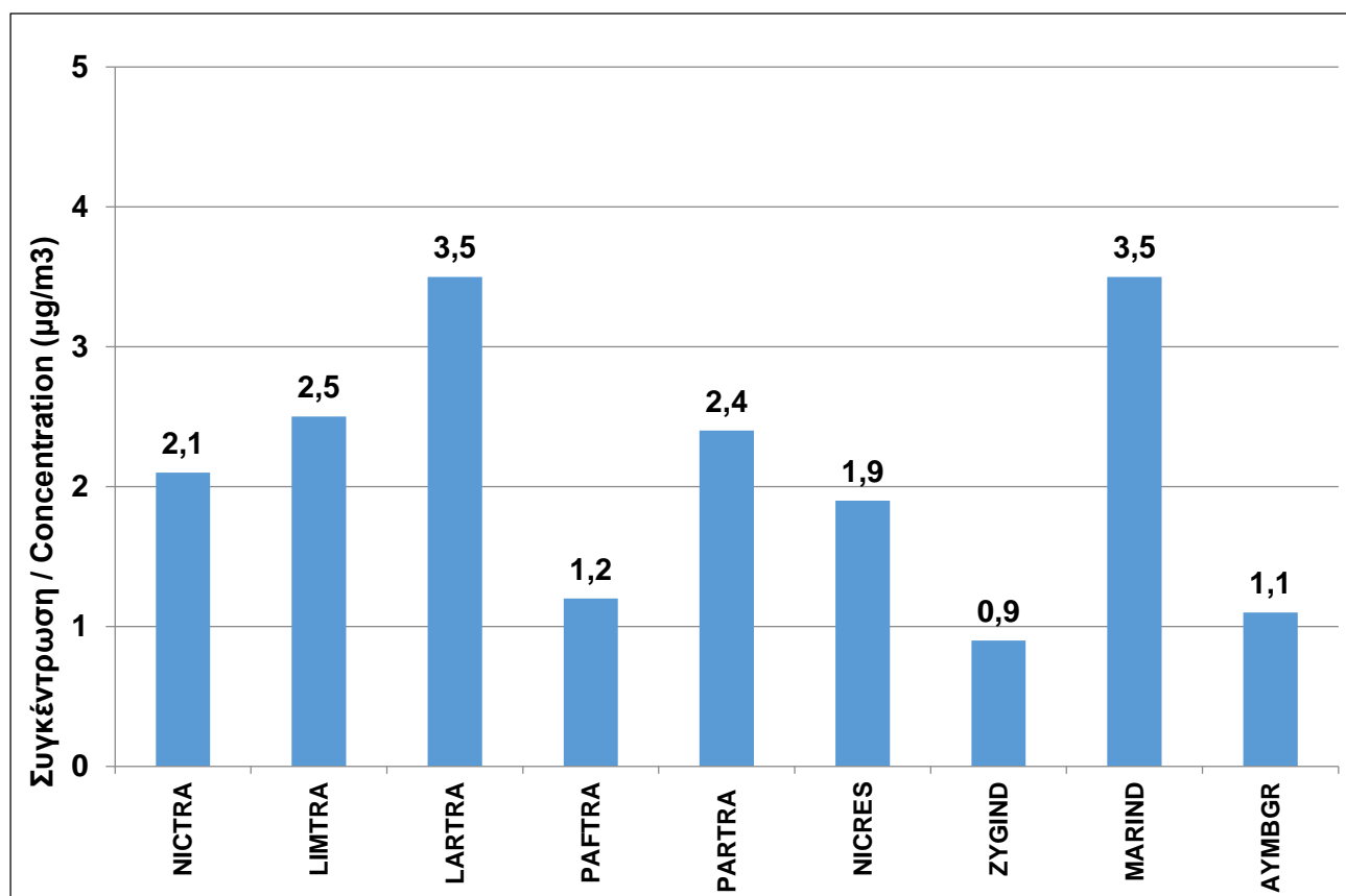
Σχήμα 6: Ετήσιοι μέσοι όροι \text{SO}_2 στους Σταθμούς Παρακολούθησης Ποιότητας Αέρα για το έτος 2018. Figure 6: \text{SO}_2 annual mean concentration in Air Quality Monitoring Stations for the year 2018.
