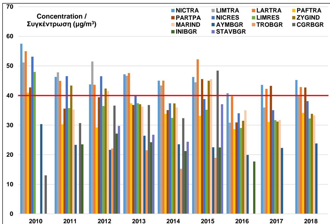
Σχήμα 11: Ετήσιοι μέσοι όροι ΑΣ 10 στους Σταθμούς Παρακολούθησης Ποιότητας Αέρα για την περίοδο 2010-2018 (Ετήσια οριακή τιμή: 40 \mu\text{g}/\text{m}^3 ).
