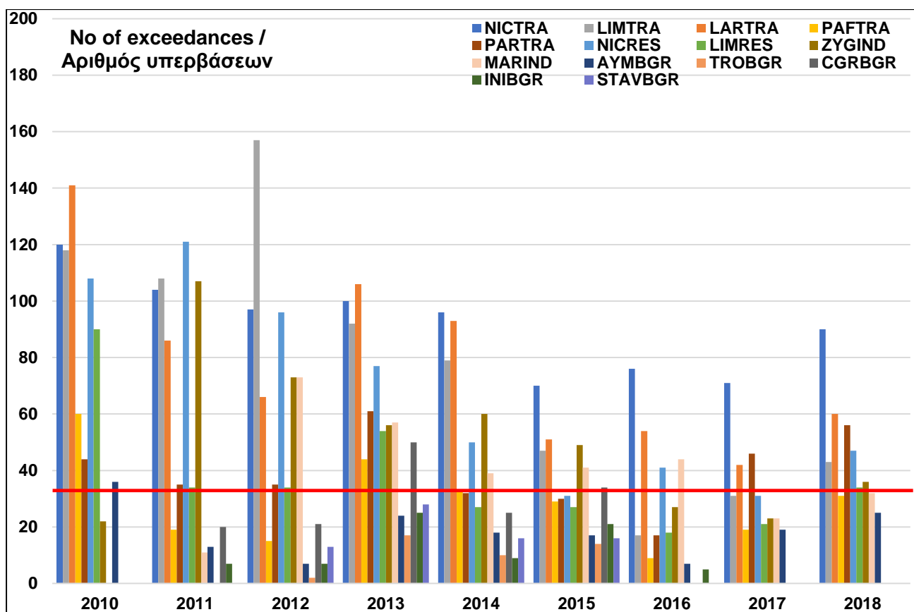
Σχήμα 12: Αριθμός υπερβάσεων ανά έτος της ημερήσιας οριακής τιμής ΑΣ_{10} στους Σταθμούς Παρακολούθησης Ποιότητας Αέρα για την περίοδο 2010-2018 (Αριθμός επιτρεπτών υπερβάσεων: 35).
