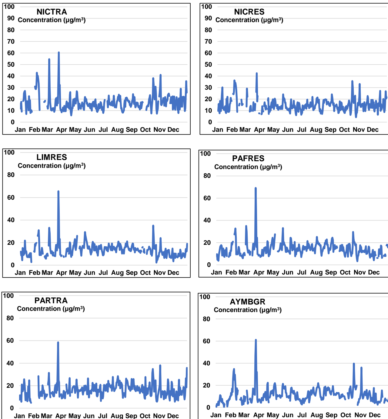
Σχήμα 15: Ημερήσια συγκέντρωση Αιωρούμενων Σωματιδίων με αεροδυναμική διάμετρο 2,5 µm (ΑΣ 2,5 ) στους Σταθμούς Παρακολούθησης Ποιότητας Αέρα για το έτος 2018.
