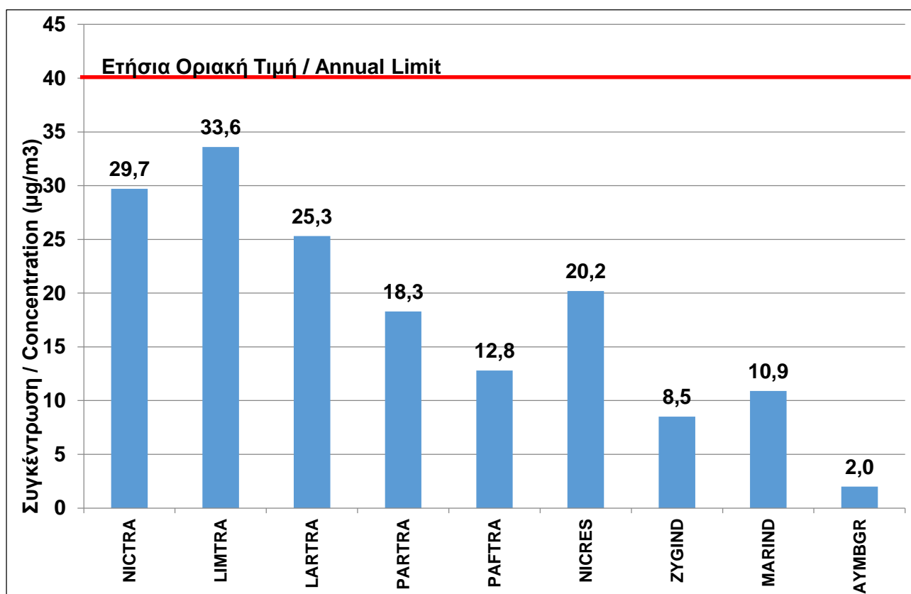
Σχήμα 4: Ετήσιοι μέσοι όροι \text{NO}_2 στους Σταθμούς Παρακολούθησης Ποιότητας Αέρα για το έτος 2018. Figure 4: \text{NO}_2 annual mean concentration in Air Quality Monitoring Stations for the year 2018.
