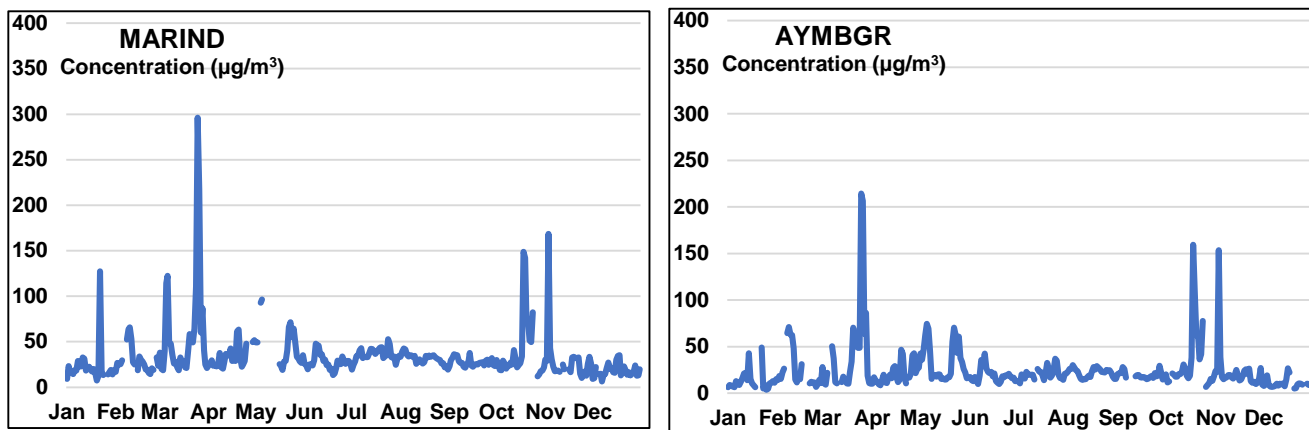
Σχήμα 14: Ημερήσια συγκέντρωση Αιωρούμενων Σωματιδίων με αεροδυναμική διάμετρο 10 µm (ΑΣ 10 ) στους Σταθμούς Παρακολούθησης Ποιότητας Αέρα για το έτος 2018 (Ημερήσια οριακή τιμή: 50 µg/m 3 ).
